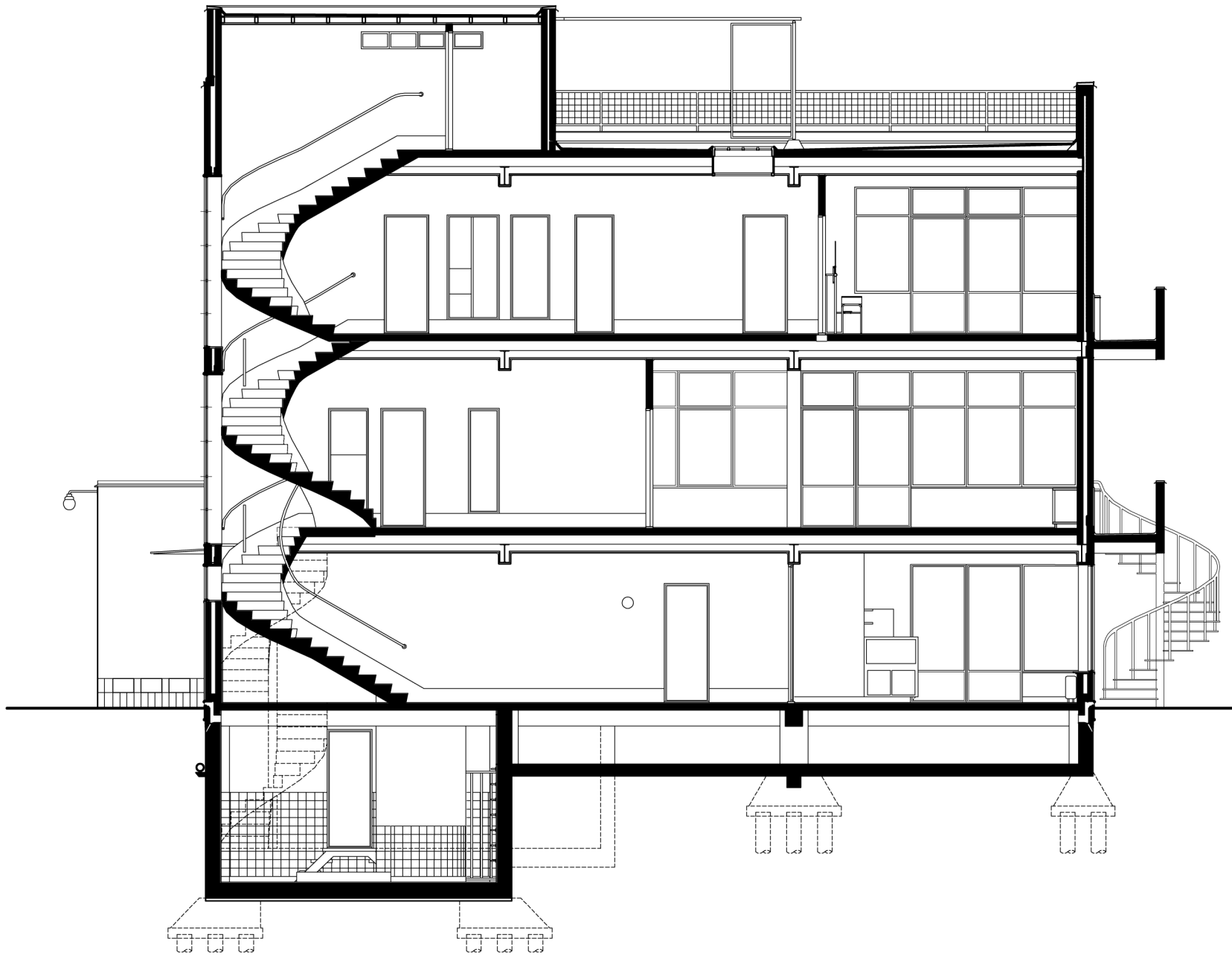
LANGSDOORSNEDE
